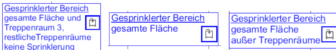
Abbildung 3: Beispiele Darstellung gesprinklerte / mit Gas gelöschte Bereiche und Löschmittelzentralen
