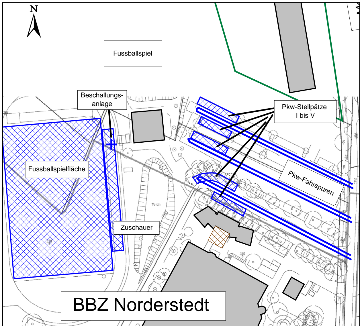
Abbildung 12. Fußballpunkt- und trainingsspiele, Lageplan der Quellenn, Maßstab 1 : 1.500.
