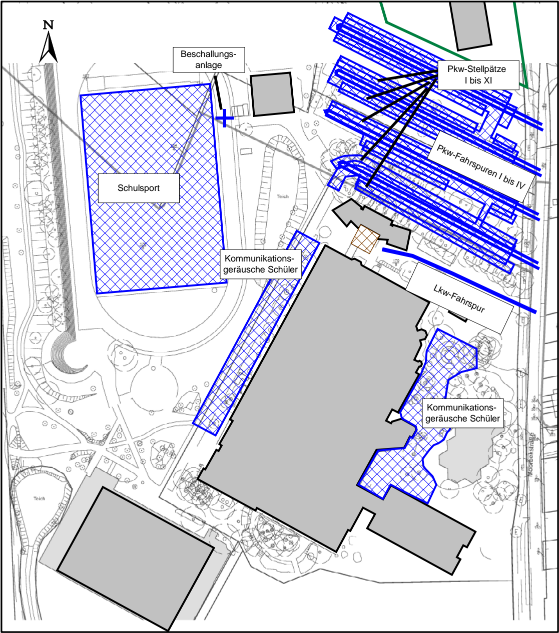
Abbildung 14. Schulbetrieb, Lageplan der Quellen, Maßstab 1 : 2.000.
