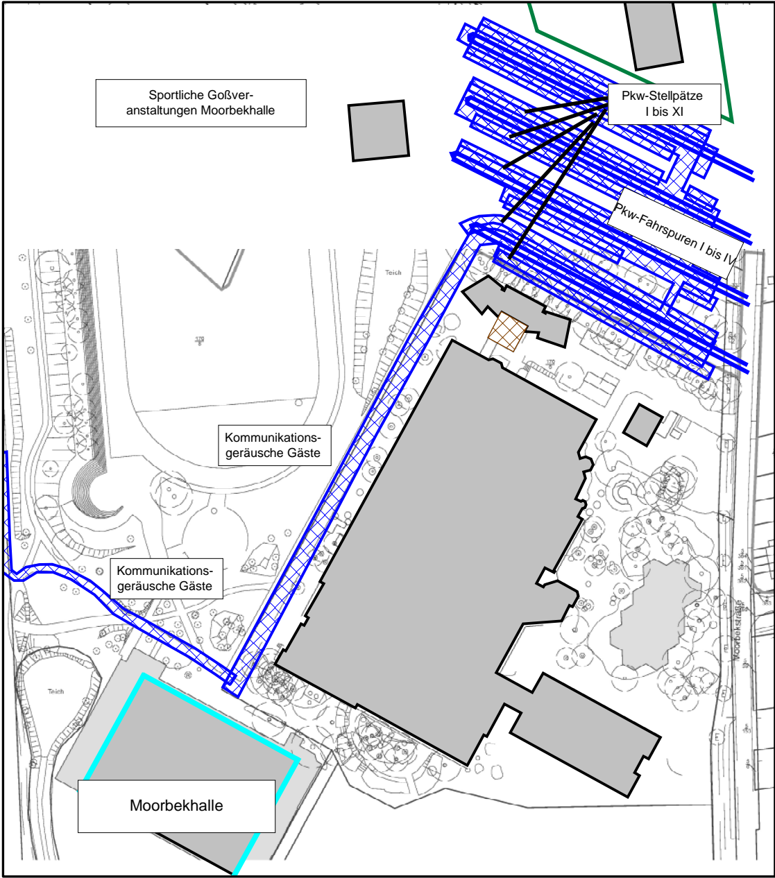
Abbildung 13. Sportliche Großveranstaltungen, Lageplan der Quellen, Maßstab 1 : 2.000.
